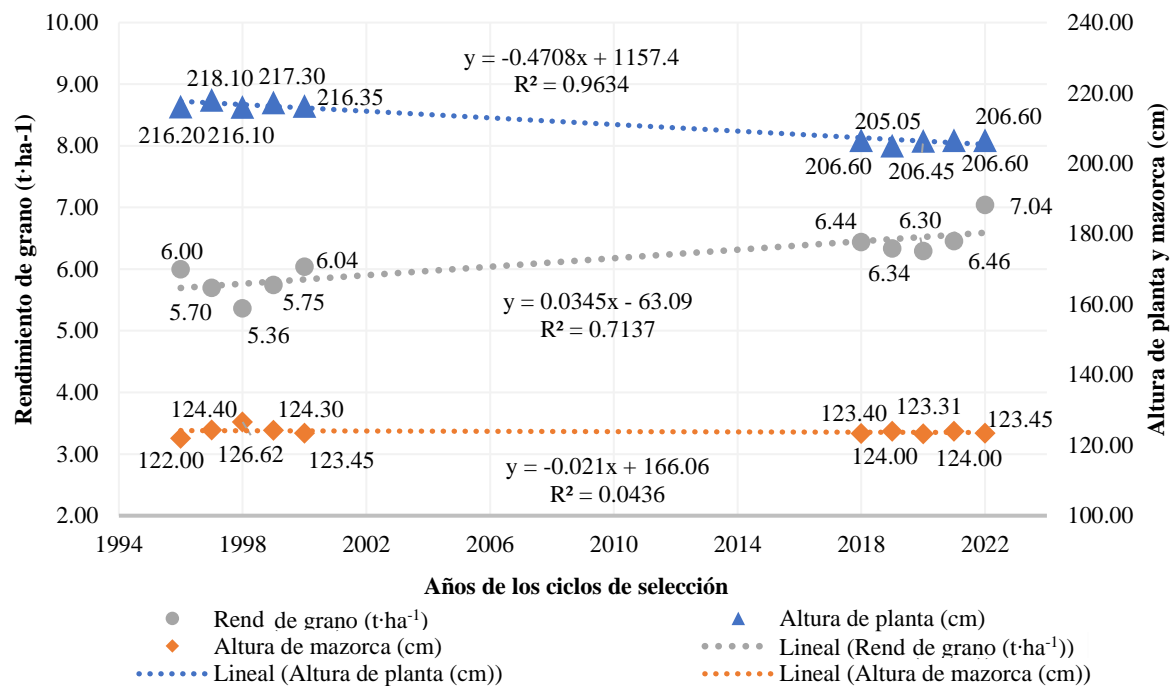
Figura 2. Dispersión de los valores tendencia lineal entre los valores de los dos periodos de selección 1996 a 2000 y 2018 a 2022 de la variedad Marginal 28T
